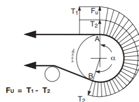
Fig. 5. Variazione della tensione attorno al tamburo motore
